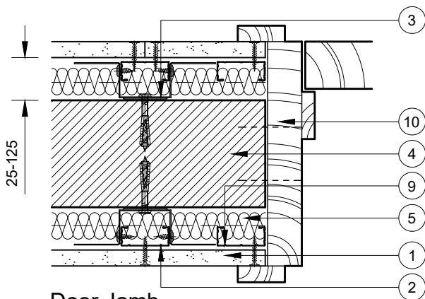
Door Jamb
